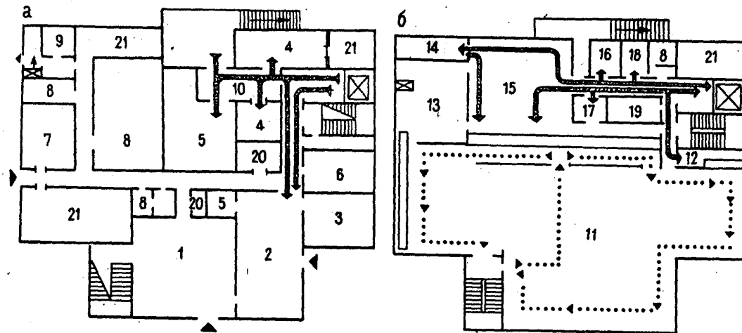
Рис. 5. Схема функционально-технологической структуры столовой на 200 мест, работающей на полуфабрикатах высокой степени готовности для зон отдыха
