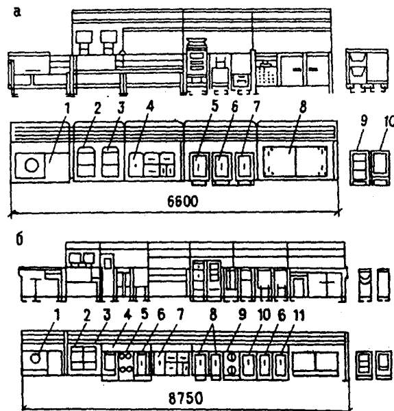
Рис. 4. Примеры комплектации линий самообслуживания
