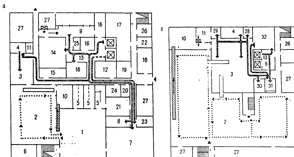
Рис. 9. Схема планировочной функционально-технологической структуры столовой на 500 мест на полуфабрикатах для высших учебных заведений
