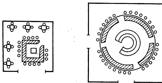
Рис. 12. Принципы размещения и композиционные решения эстрад, мест для танцев (а); барных стоек (б)
