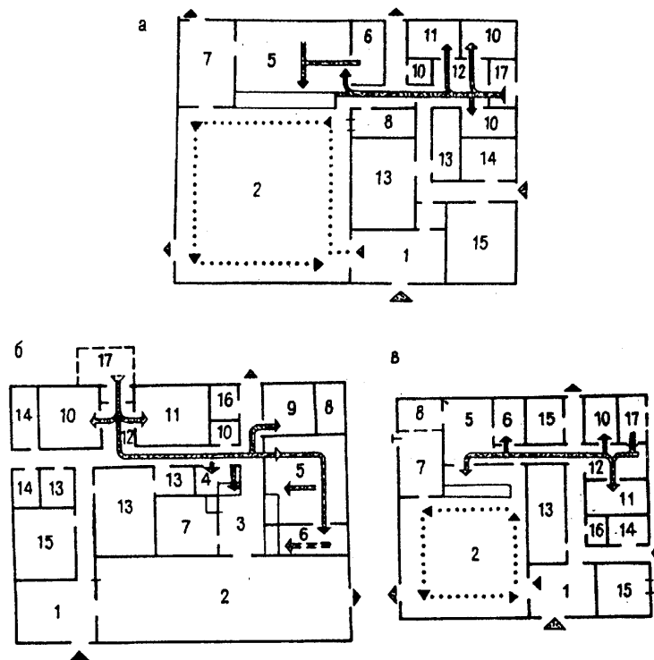
Рис. 8. Схема планировочной функционально-технологической структуры предприятий
