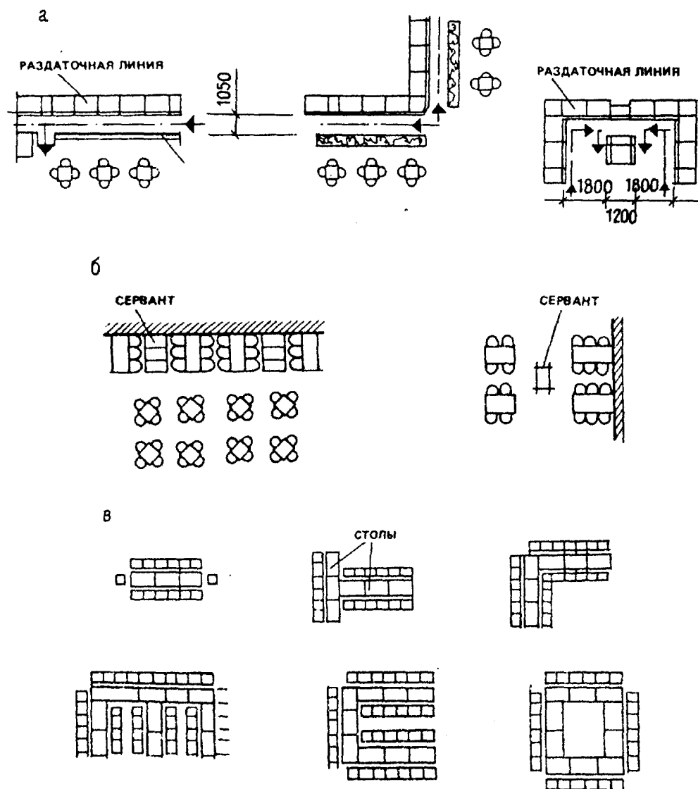
Рис. 11. Функциональные зоны в обеденных и банкетных залах
