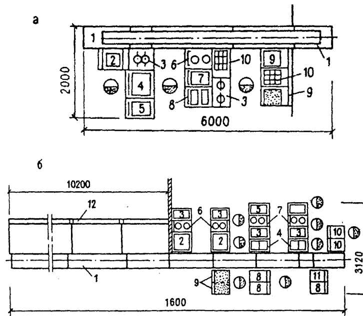
Рис. 10 Технологическое оборудование для отпуска комплексных обедов
