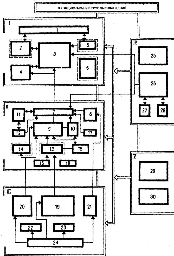
Рис. 2. Схема взаимосвязи функциональных групп помещений доготовочных предприятий общественного питания обслуживаемых официантами
